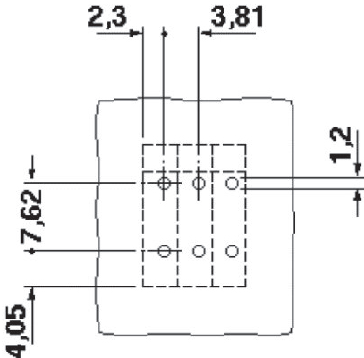
Esquema de pinagem/Geometria de pino de solda
