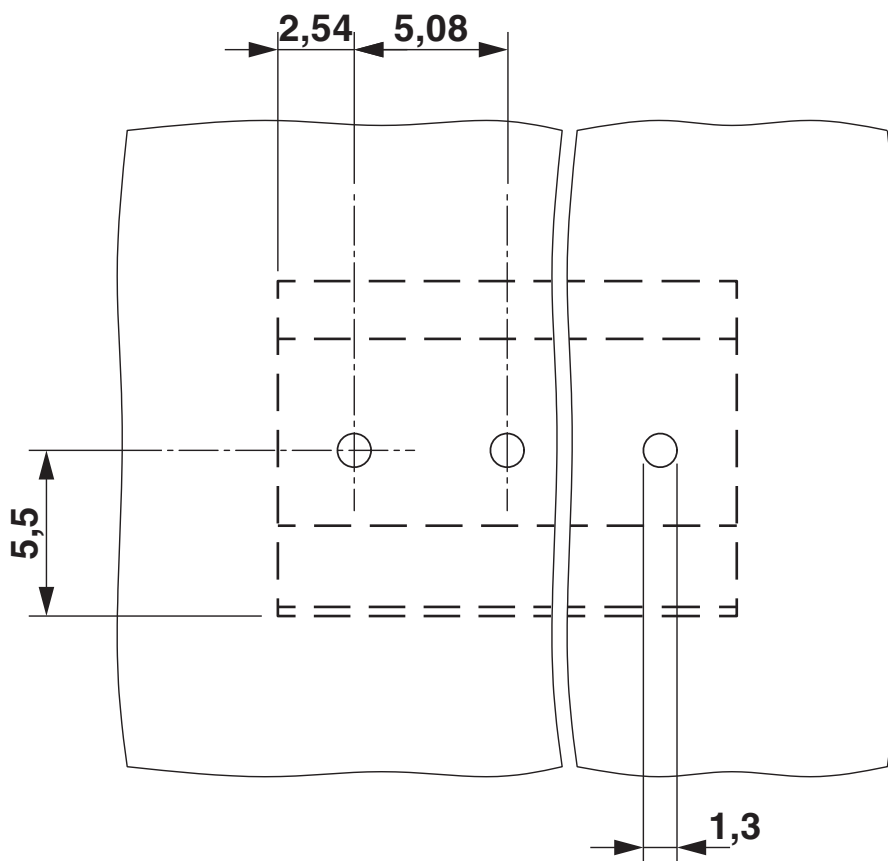
Esquema de pinagem/Geometria de pino de solda
