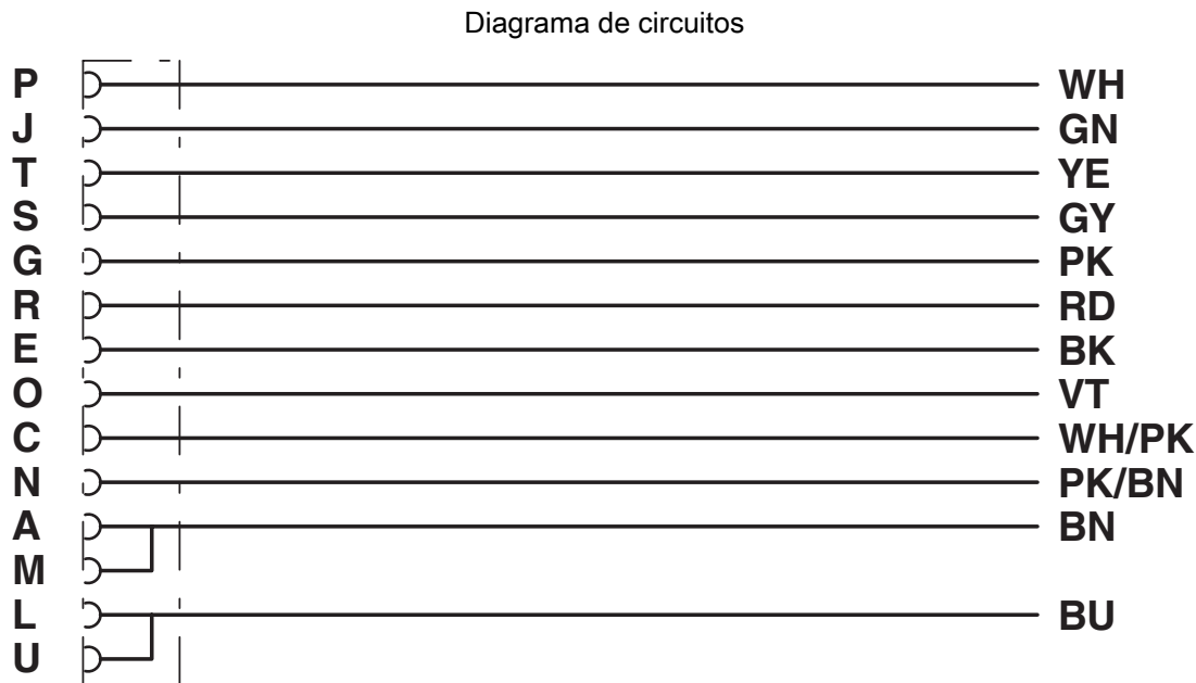
Alocação de conexão do soquete M16
