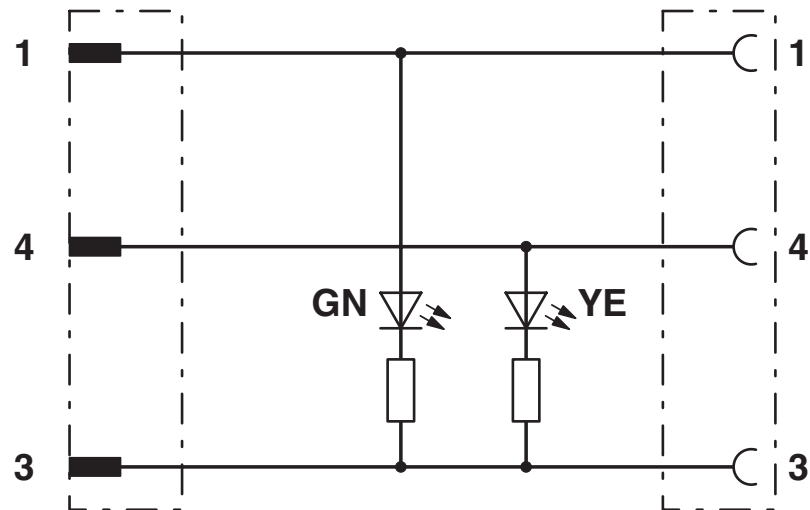
Diagrama de circuitos
