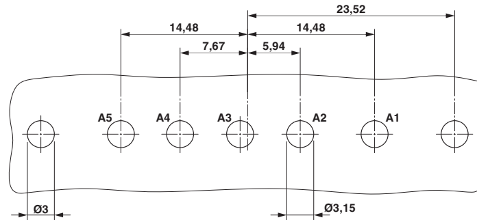
Esquema de pinagem/Geometria de pino de solda
