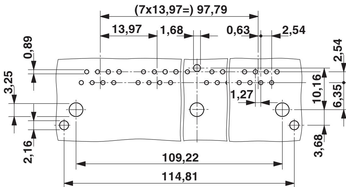
Esquema de perfuração
