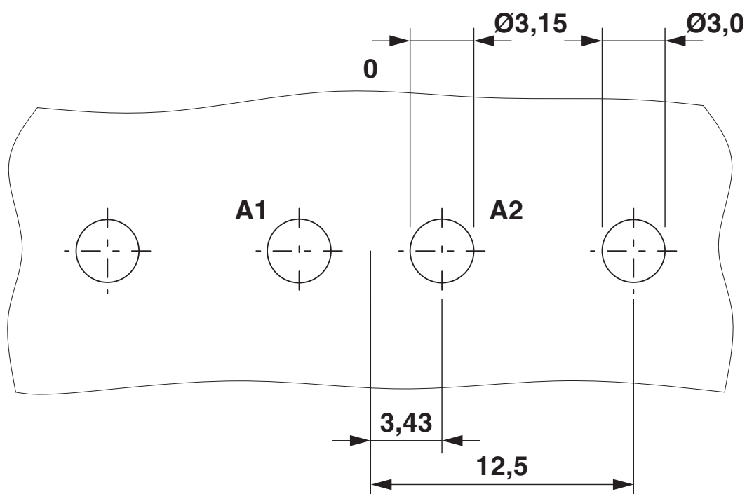
Esquema de pinagem/Geometria de pino de solda
