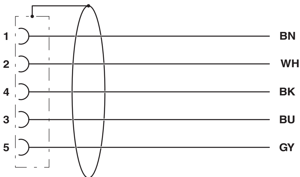
Esquema de ligação do soquete M12
