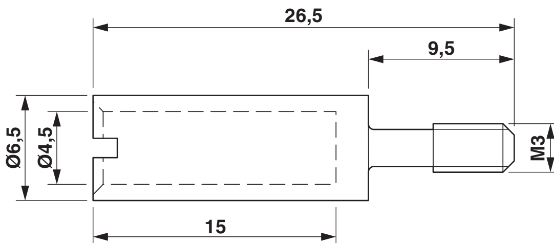
Desenho com dimensões
