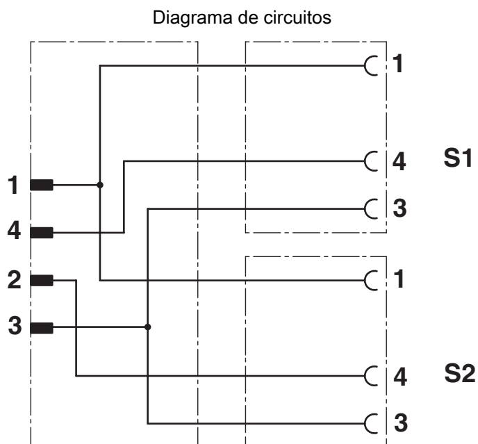
Alocação de conexão do plugue M12 e dos soquetes M8
