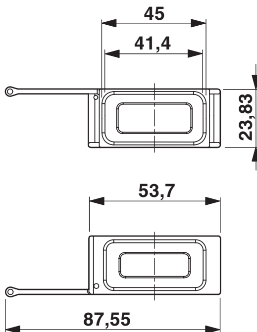
Desenho de medidas
