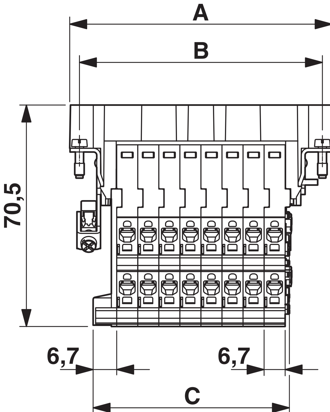
Desenho de medidas
