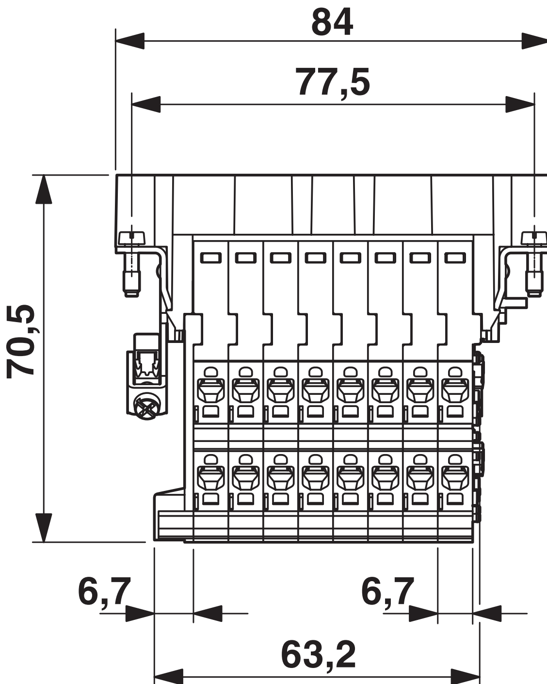
Desenho com dimensões
