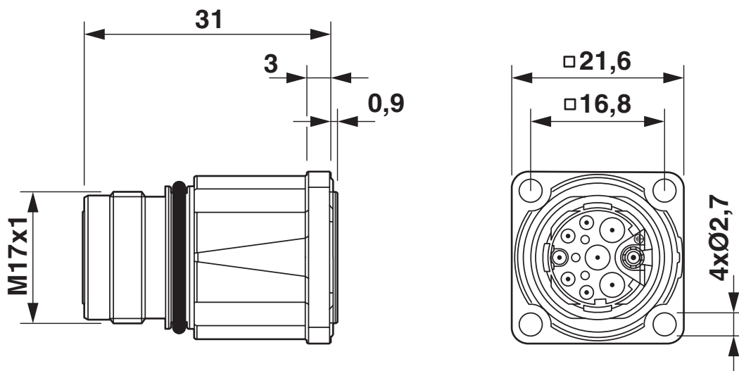
Desenho com dimensões
