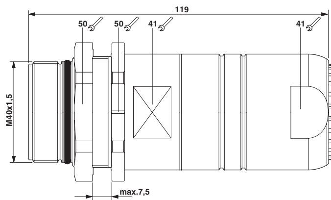
Desenho de medidas
