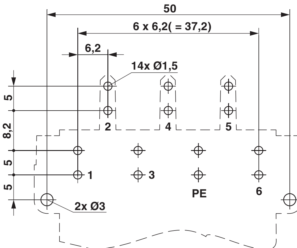
Esquema de pinagem: DC-...PCB-90
