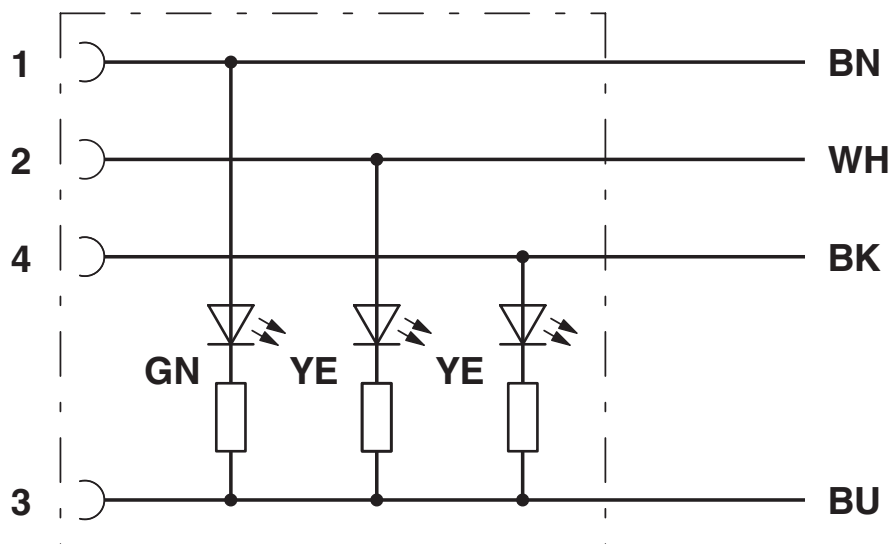
Alocação de conexão do plugue M12 / soquetes com LED
