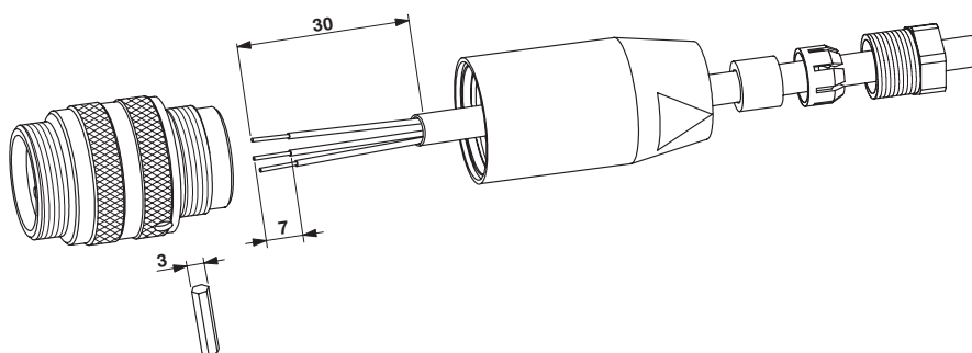
Desenho funcional
