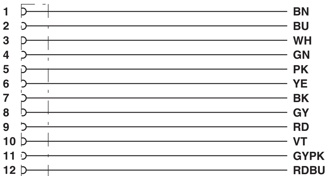
Esquema de ligação do soquete M12
