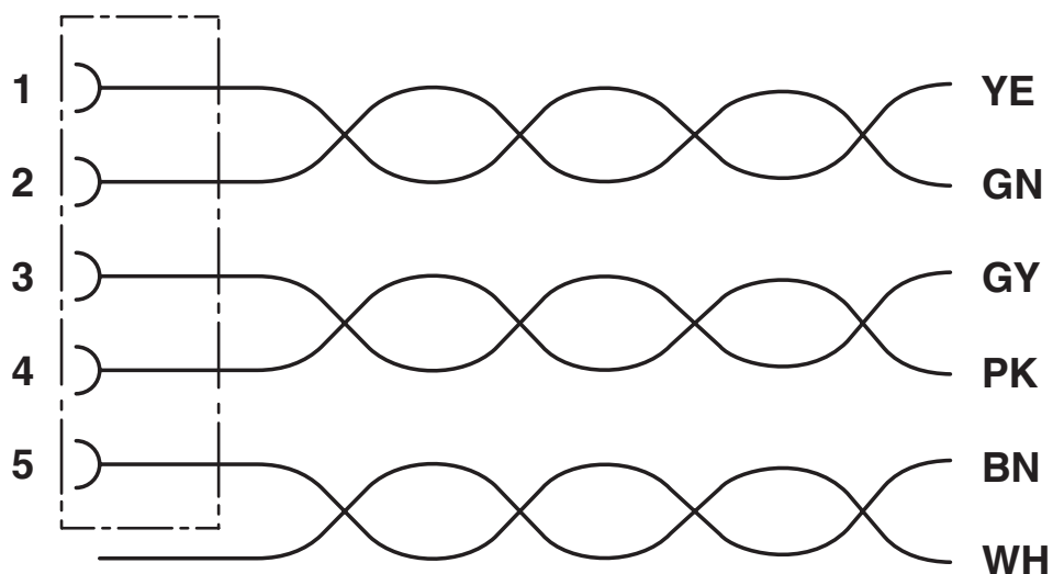
Diagrama de circuitos
