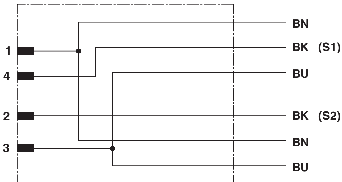
Esquema elétrico do plugue conector M12 Y
