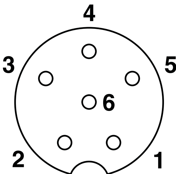
Imagem com pólos soquete M8, 6 pólos, vista lado do soquete
