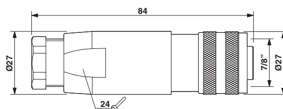
Desenho de medidas
