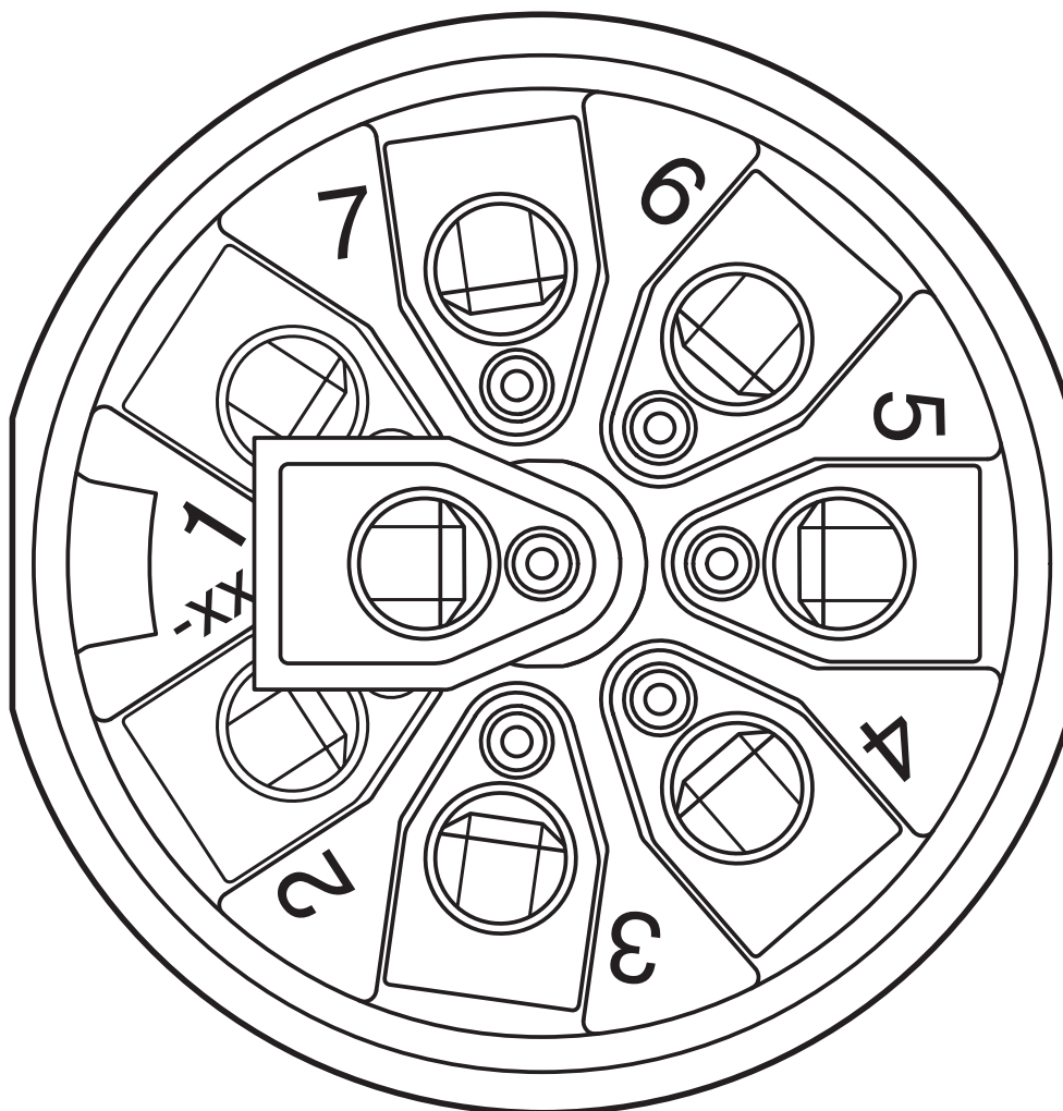
Lado de conexão do cabo M12 (conexão a parafuso)
