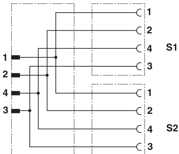
Alocação de conexão do plugue Y M12 e dos soquetes M12
