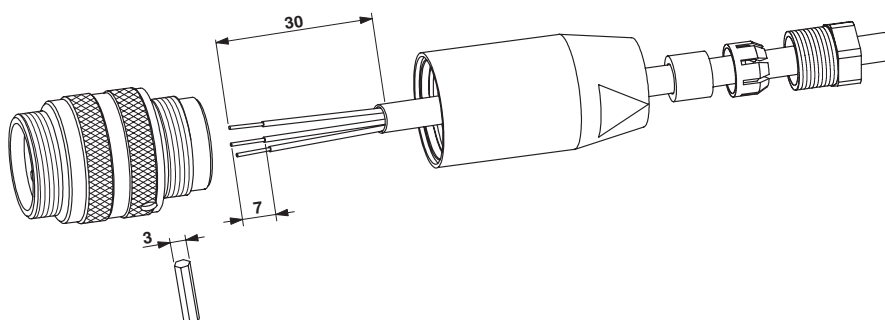
Desenho funcional
