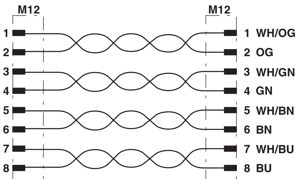
Alocação de contato dos conectores M12
