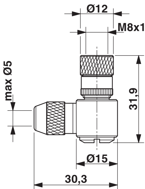
Desenho de medidas
