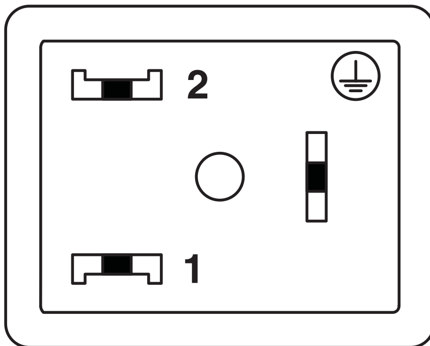
Imagem com pólos conector para válvula, formato B
