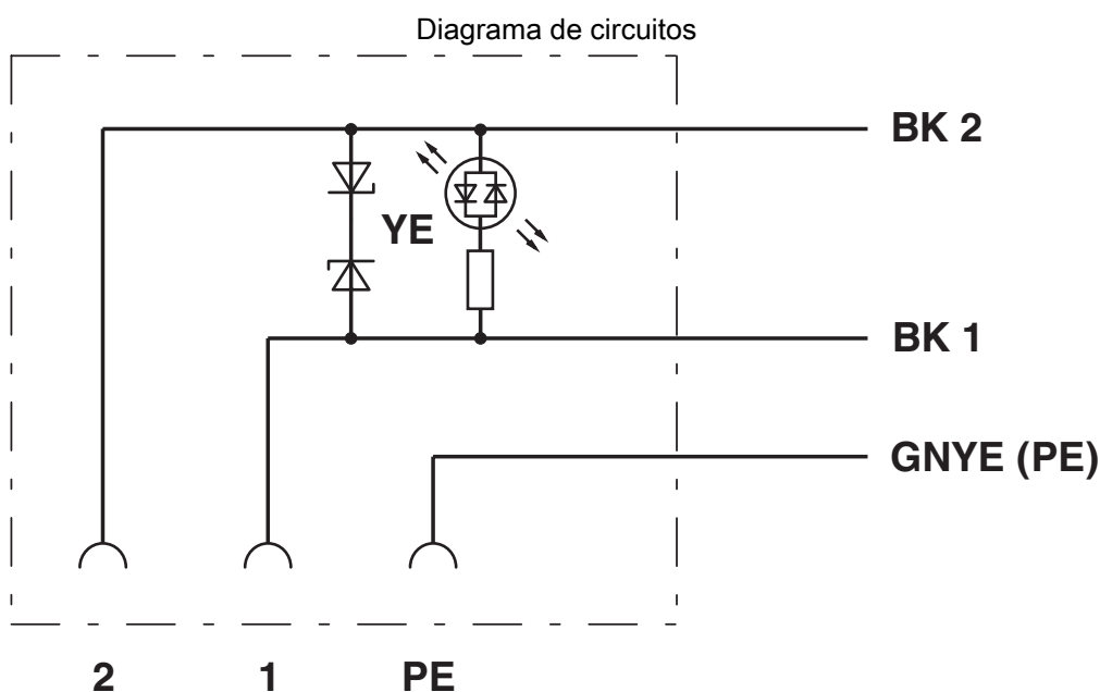
Alocação de conexão do conector para válvula
