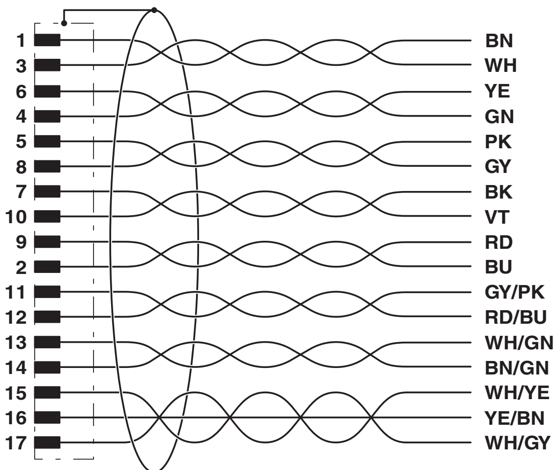
Esquema de ligação do conector M12
