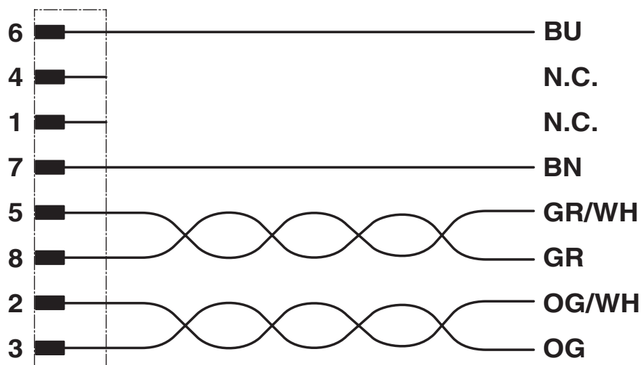
Esquema de ligação do conector M12
