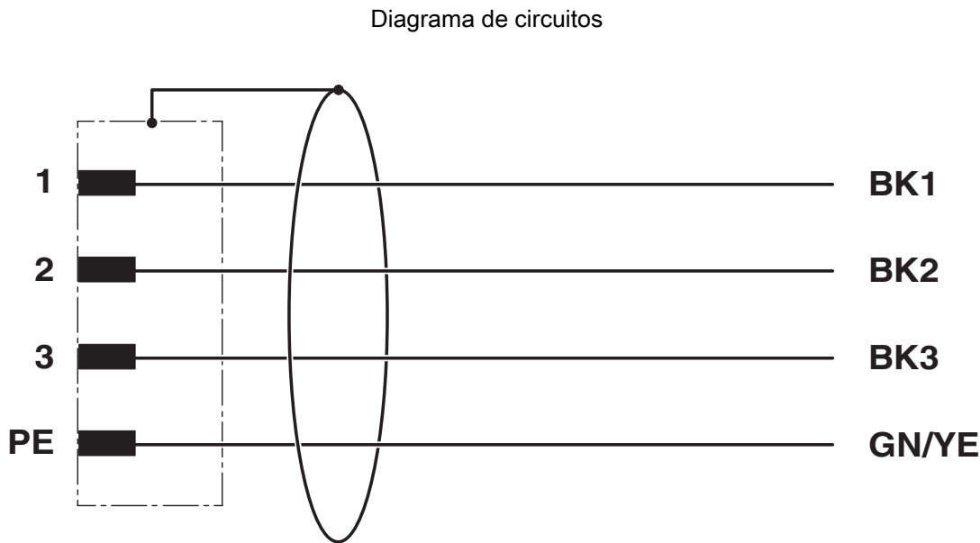
Esquema de ligação do conector M12
