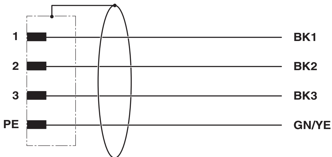
Esquema de ligação do conector M12
