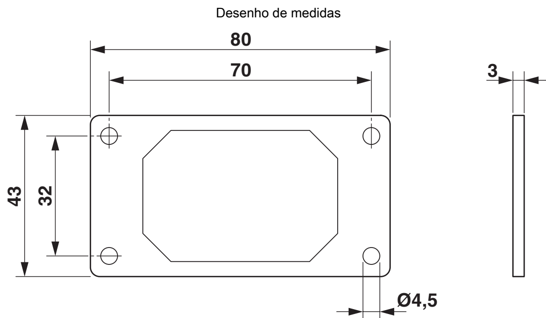
Desenho com dimensões
