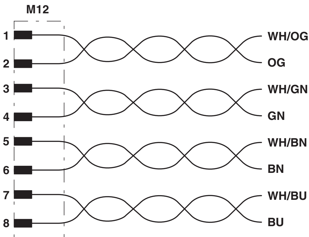
Esquema de ligação do conector M12
