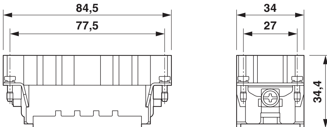
Desenho com dimensões
