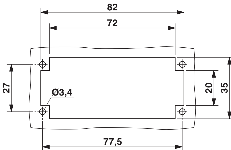
Recorte de montagem para aplicação sem caixa
