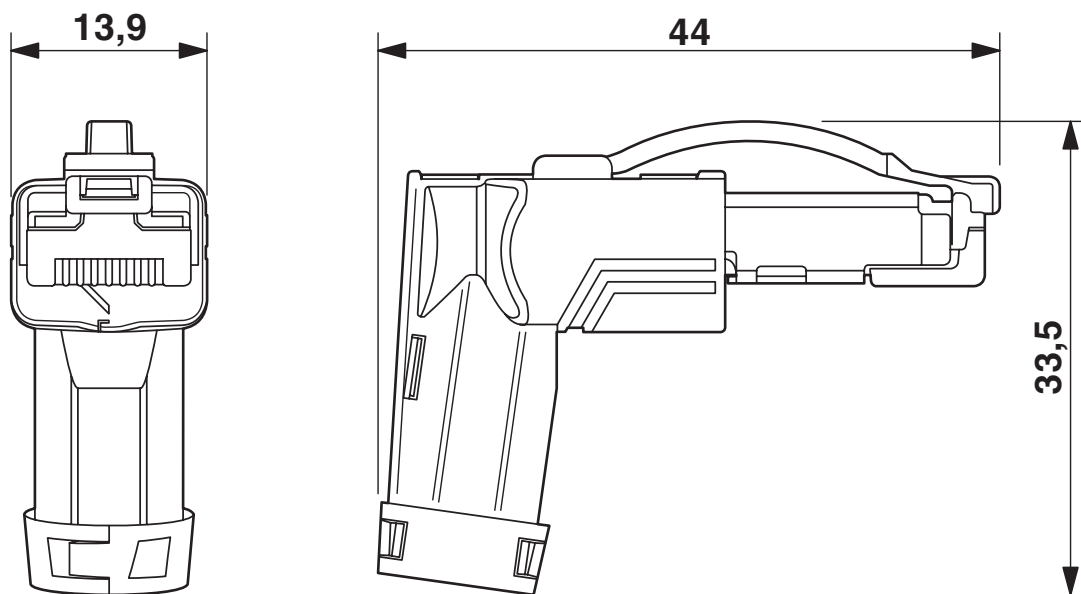
Conector de encaixe RJ45, IP20, angular
