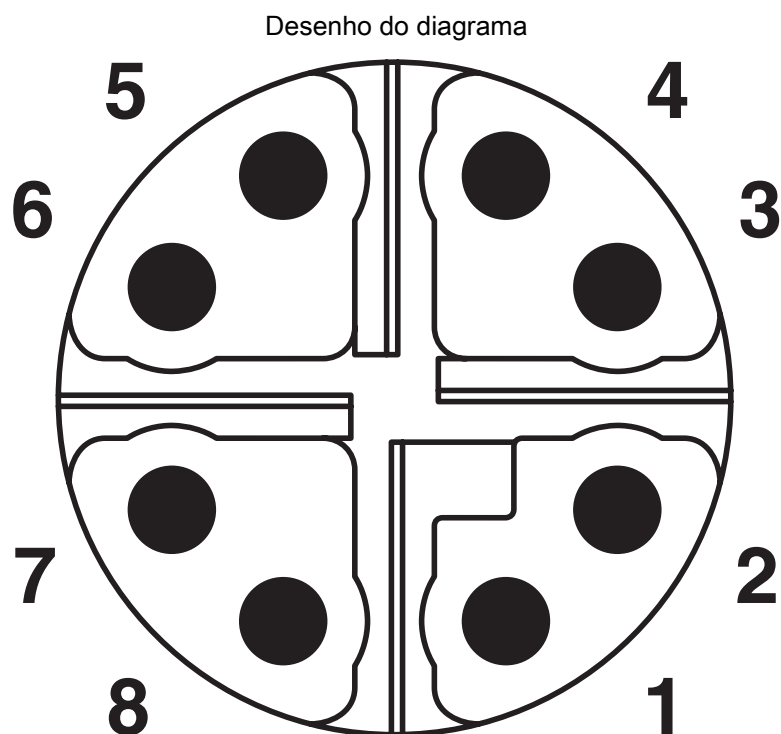
Imagem de polos Conector M12, 8 polos, codificação X, visão do lado do pino
