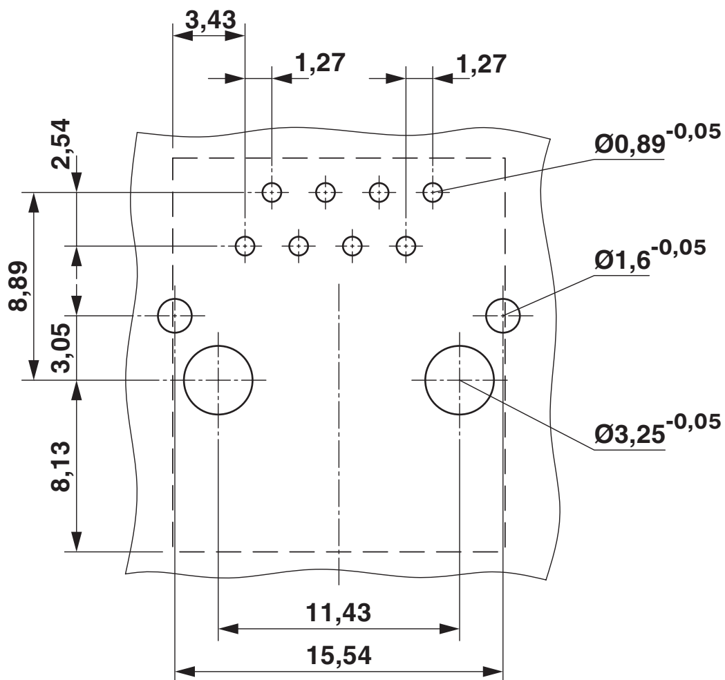
Esquema de pinagem/Geometria de pino de solda
