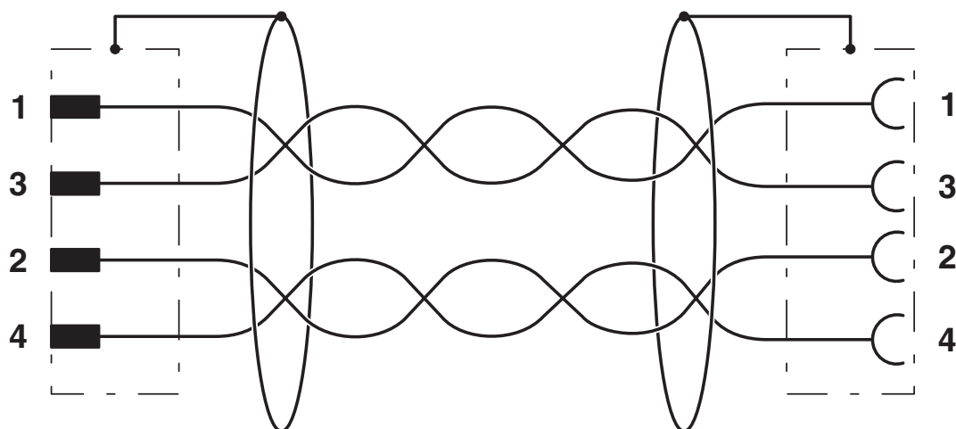
Esquema de ligação do plugue M12 e soquete M12
