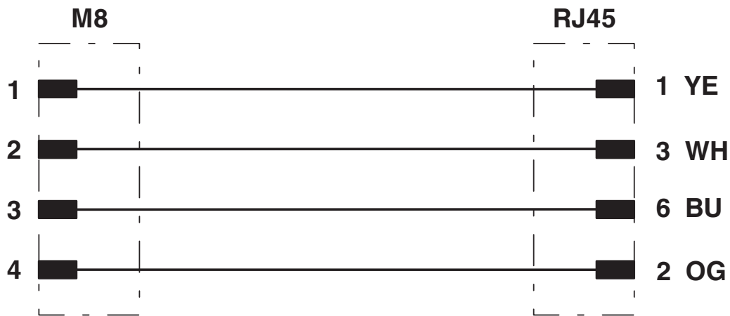
Alocação de conexão dos conectores M8 e RJ45
