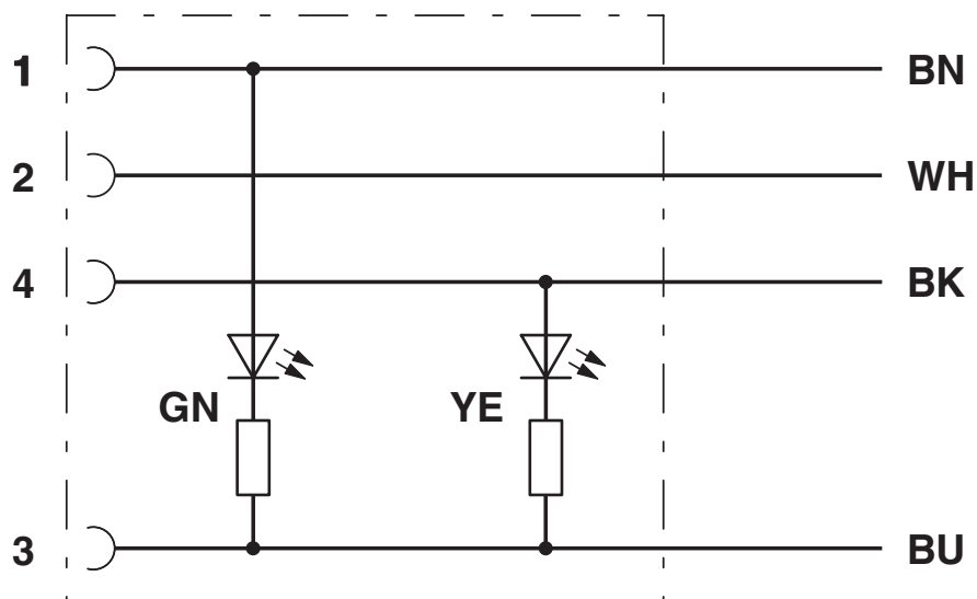
Alocação de conexão do soquete M8 com LED
