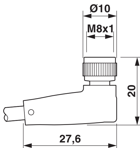
Desenho de medidas
