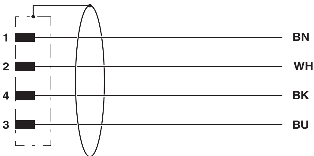
Alocação de contato dos conectores M12
