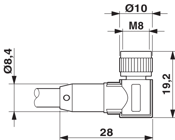
Desenho de medidas
