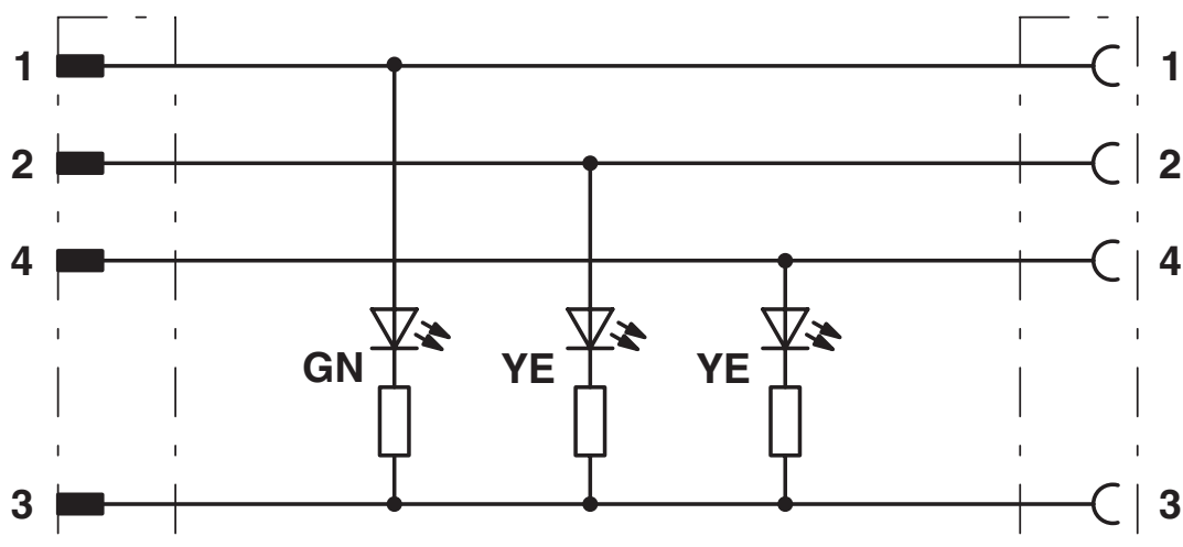
Esquema de ligação do plugue M12 e do soquete M12
