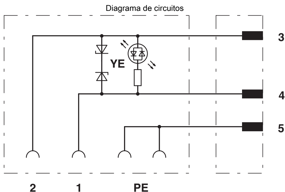
Alocação da conexão do plugue M12 e do plugue da ventoinha
