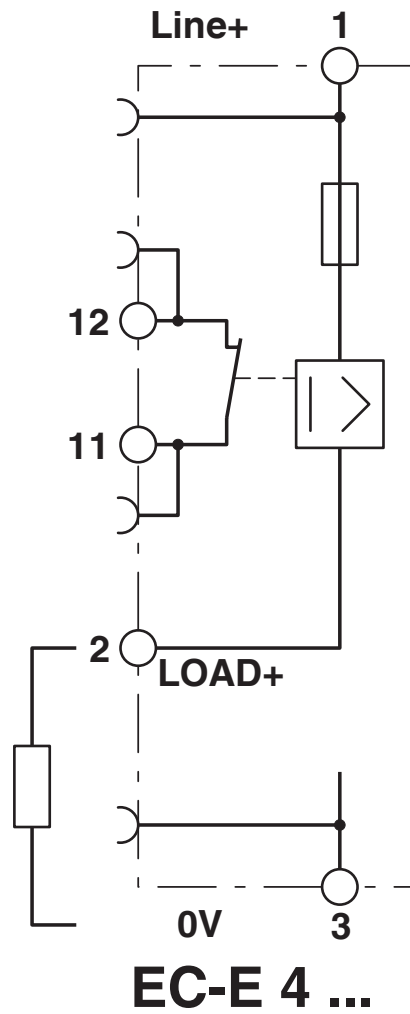
Diagrama de circuitos
