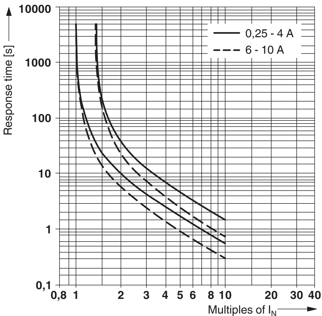
Curva característica de disparo
