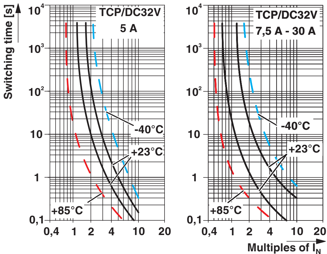
Curva característica de disparo
