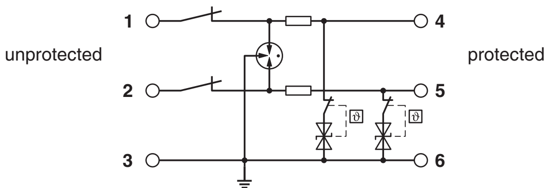
Schaltplan
